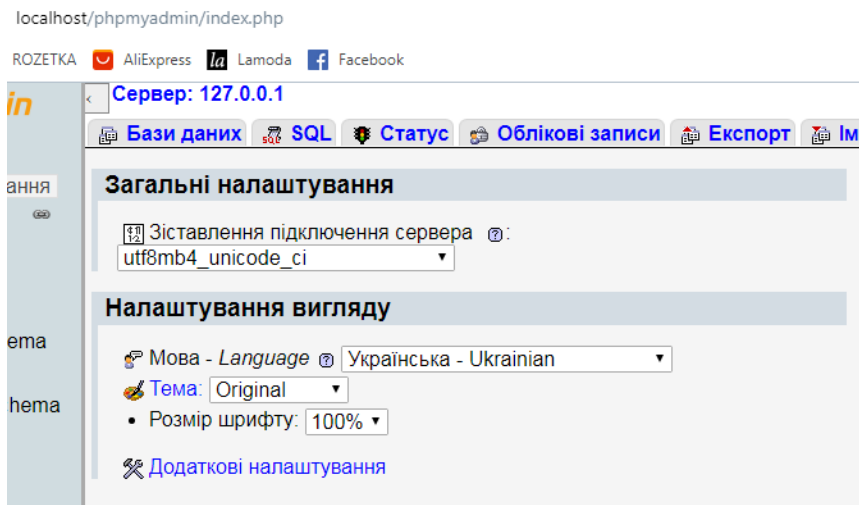
Рисунок 7.1 – Застосунок phpMyAdmin
