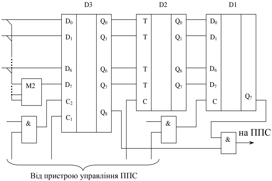
Рисунок 15 – Кодер ітеративного коду
