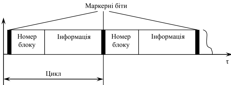
Рисунок 9 – Структура блоків при маркерному способі фазування: а) з передачею всього маркера за цикл, б) з побітною передачею
