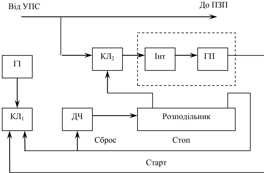
Рисунок 13 – Схема стартозастопного пристрою фазування
