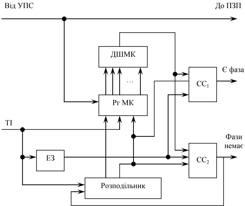
Рисунок 12 – Схема маркерного пристрою фазування з покрововим зрушенням розподільника за цикл
