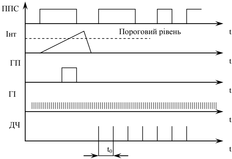
Рисунок 14 – Тимчасові діаграми роботи стартостопного ПФЦ
