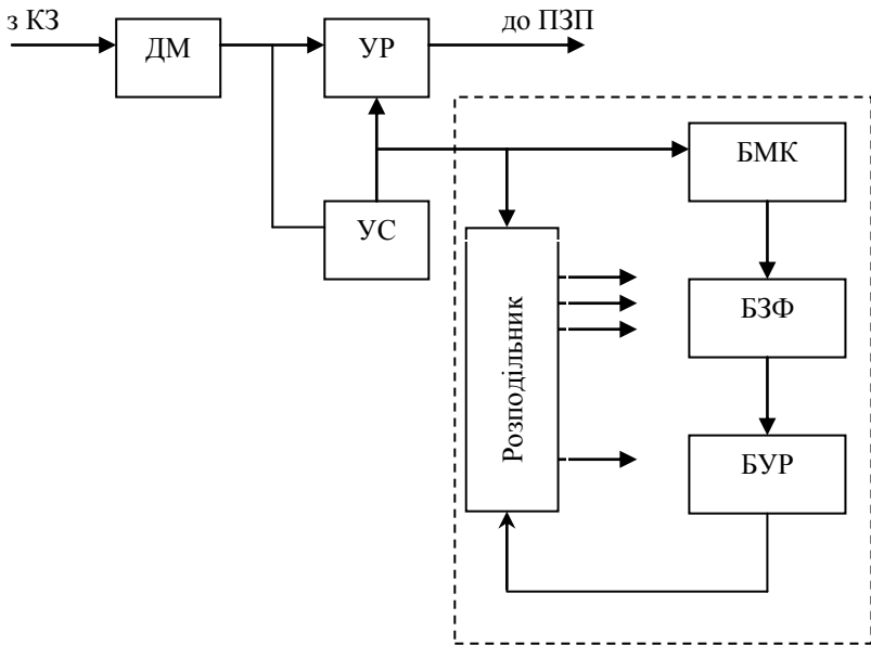
Рисунок 8 – Схема пристрою фазування по циклах
