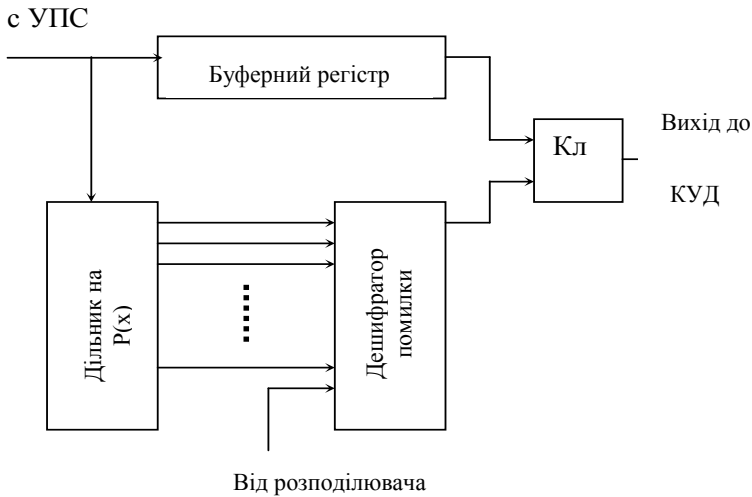
Рисунок 19 – Структурна схема декодера циклічного коду
