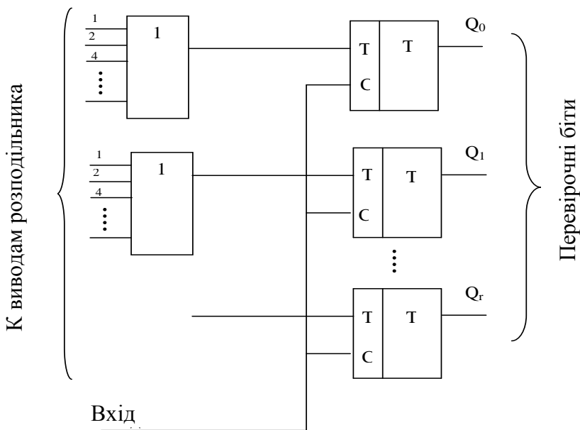
Рисунок 16 – Схема формування перевірочних елементів коду Хеммінга
