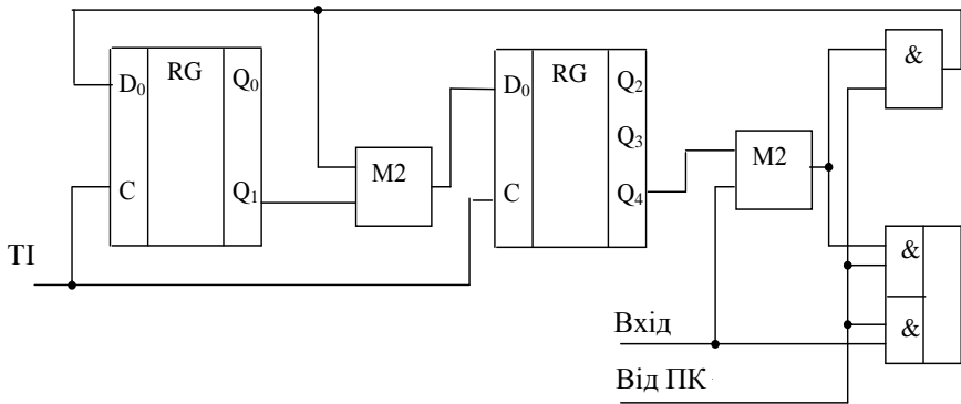
Рисунок 18 – Функціональна схема кодера циклічного коду
