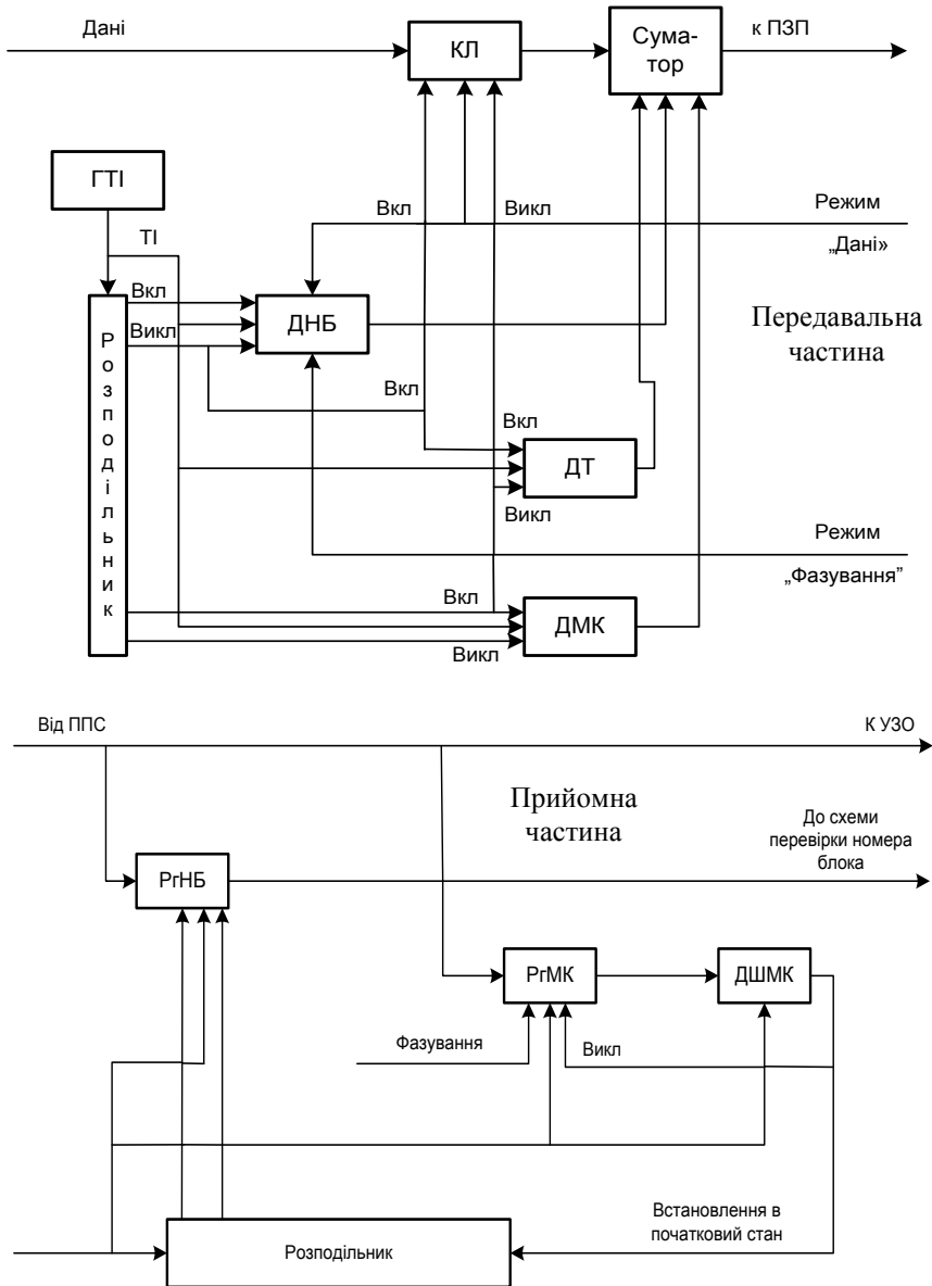
Рисунок 10 – Схеми ПФЦ для реалізації безмаркерного способу (передавальна та приймочна частини)
