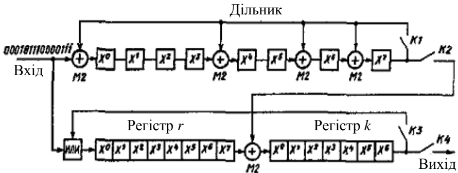
Рисунок 20 – Декодувальний пристрій
