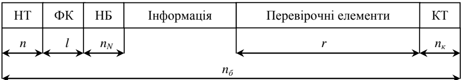
Рисунок 1 – Типовий формат блоку повідомлень
