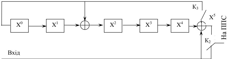
Рисунок 17 – Структурна схема пристрою, який формує циклічний код
